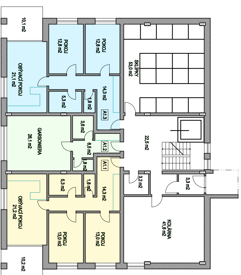
OBJEKT A1 - PŮDORYS 1.NP
