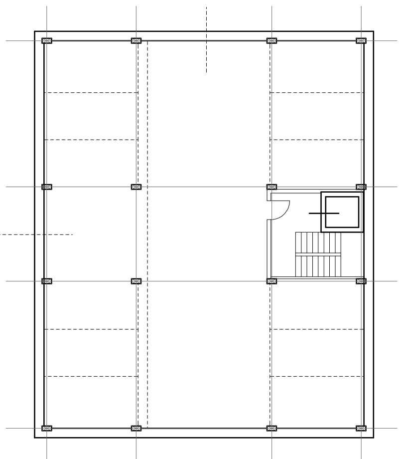
OBJEKT A1 - PŮDORYS 1.PP
