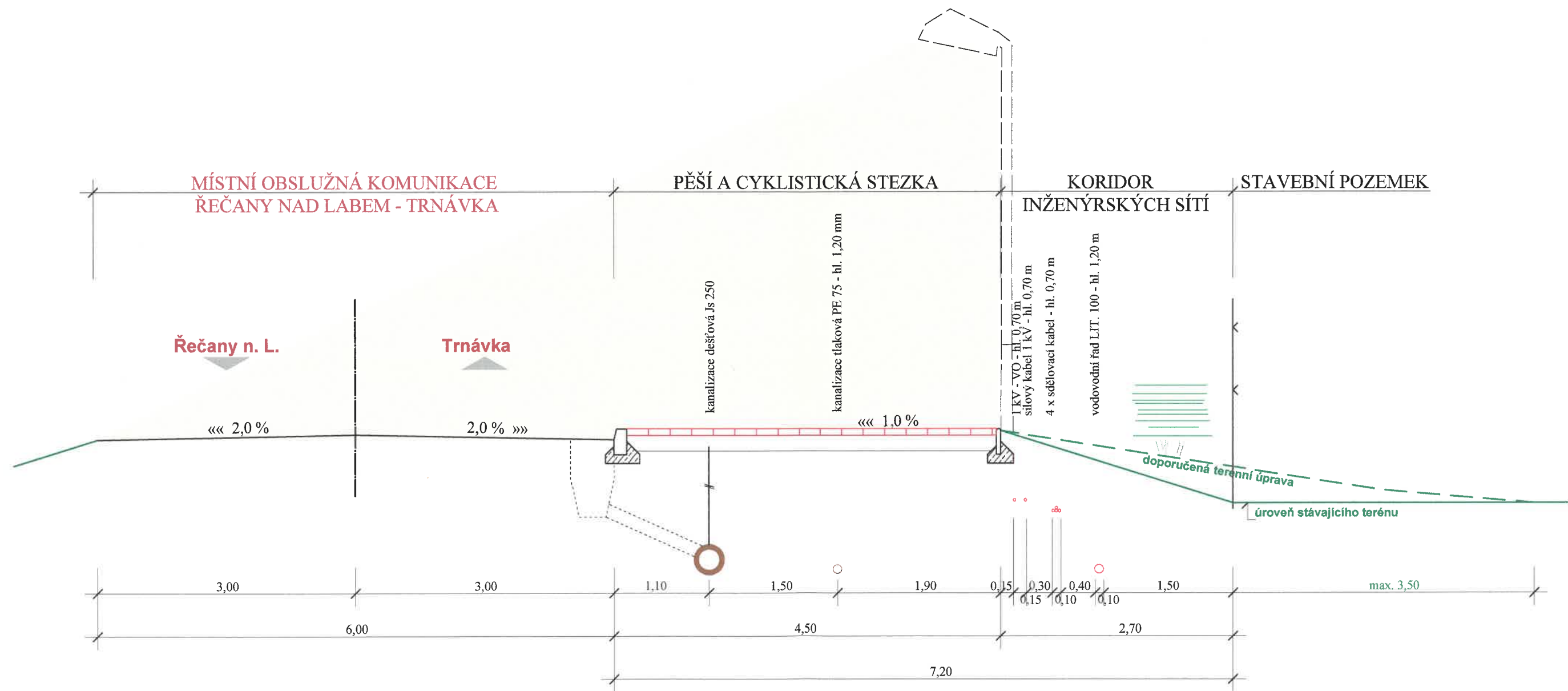
ŘEZ ULIČNÍM PROSTOREM STÁVAJÍCÍ MOK ŘEČANY NAD LABEM - TRNÁVKA 1 : 50
