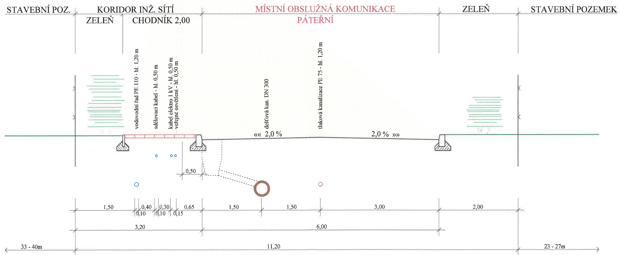
ŘEZ ULIČNÍM PROSTOREM "PÁTEŘNÍ" MOK 1 : 50
